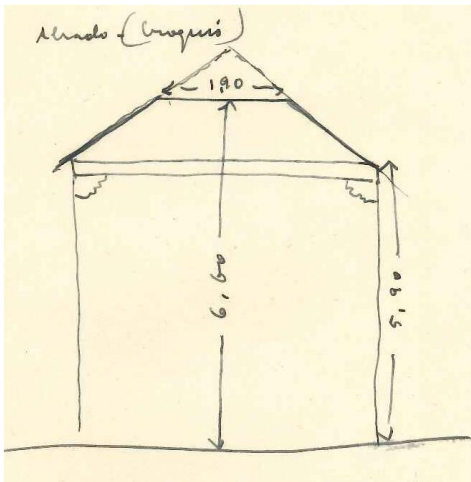
Alzado (Croquis).
